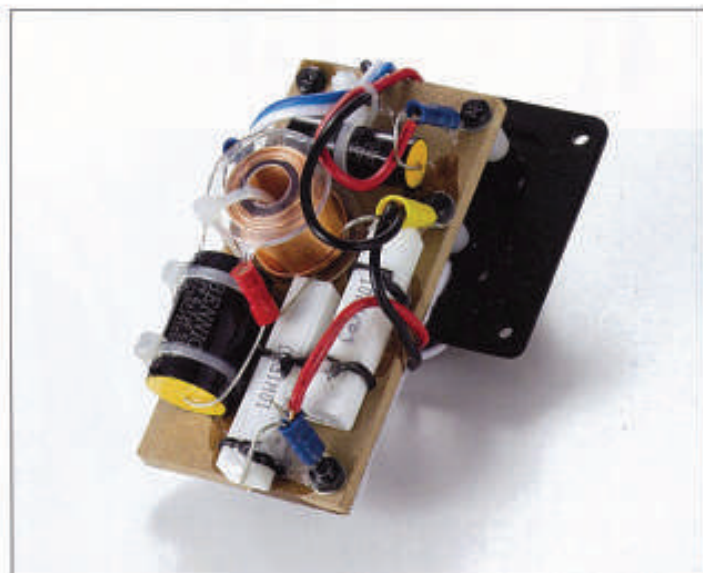
本機のネットワーク部。異種金属の接触による音質の劣化や色づけを避けるため、カシメ接続を採用。ハイパスフィルター（トゥイーター部）には高品位空芯コイルを使っている
