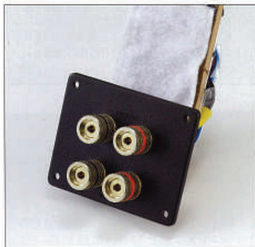
小型スピーカーでありながら、本格的なバイワイヤリング接続も可
